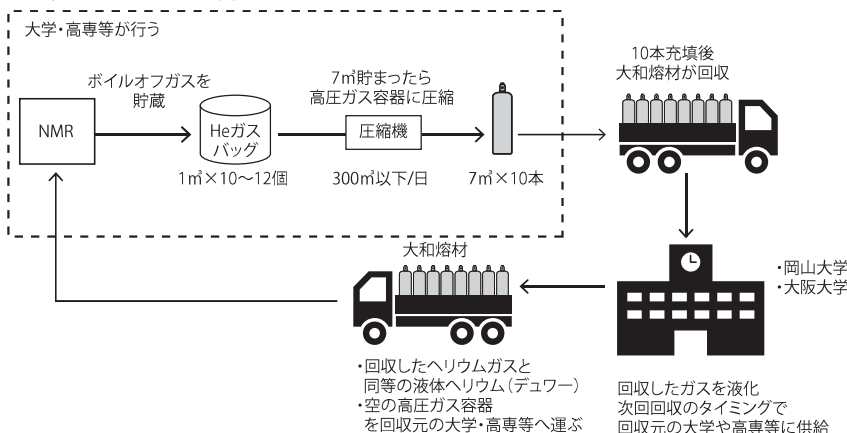
ヘリウムリサイクルフロー図
